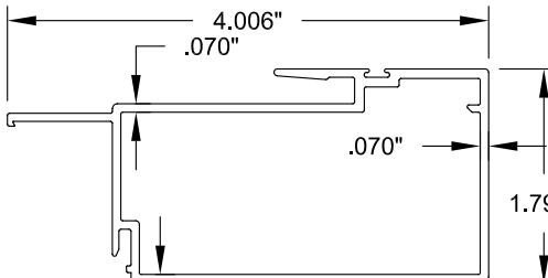
8 EXTERIOR INTERLOCK
