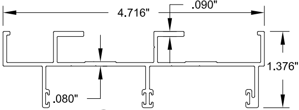
3 2-TRACK JAMB
