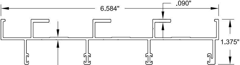
6 3-TRACK JAMB
