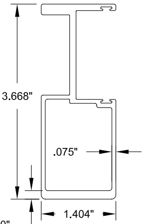
11 ASTRAGAL
